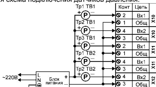
Рис. 4.4 – Пример подключения датчиков давления
