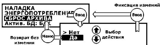
Рис. 3.12 – Сброс архива
